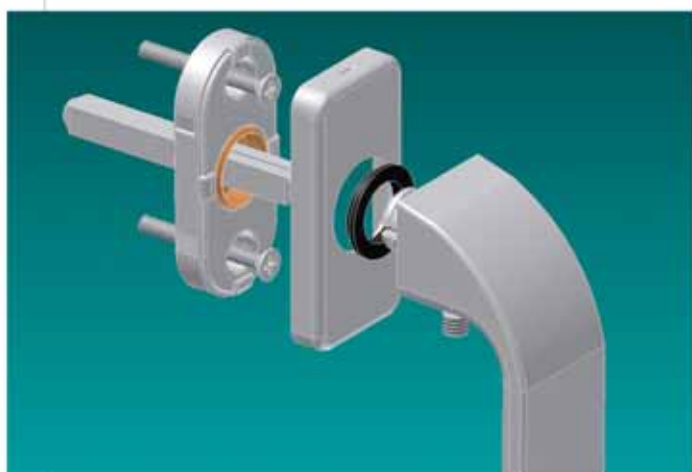
montáž okenní klika 3-4 polohová
